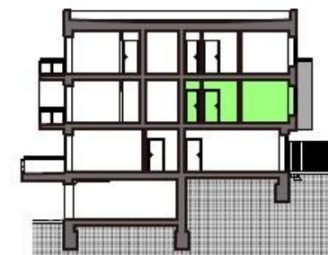
ŘEZ OBJEKTEM C1
