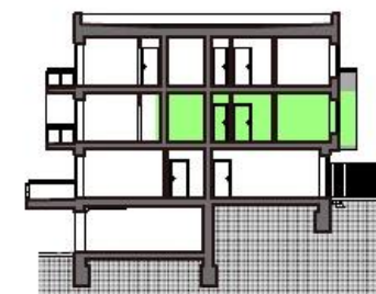
ŘEZ OBJEKTEM C1
